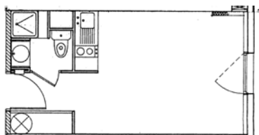
Plan studio de 19 m 2
