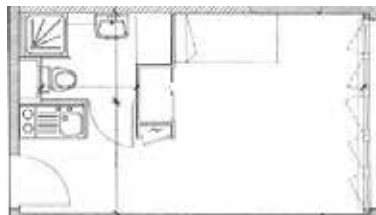
Plan studio de 22,75 m 2
